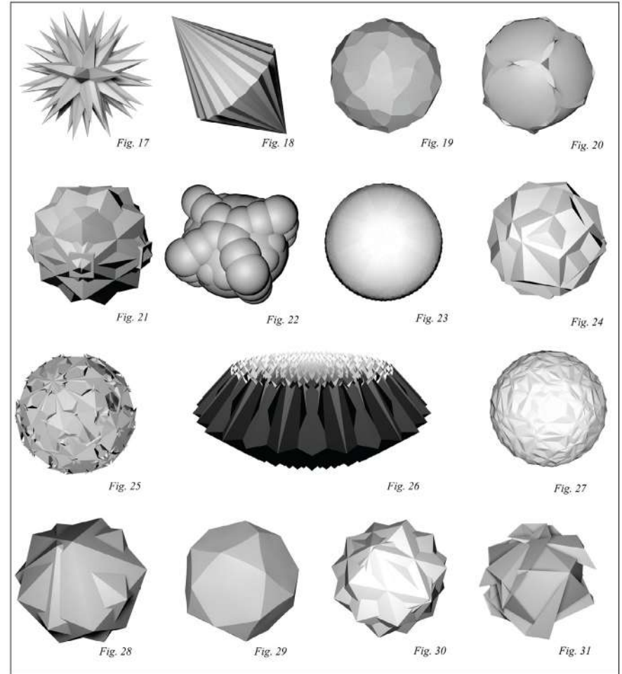
Figura 17: Betelgeuse (271°, N7°); Figura 18: Sirius (259°, S17°); Figura 19: Al Nair (28°, S47°); Figura 20: Kochab (137°, N74°); Figura 21: Gacrux (173°, S57°); Figura 22: Arcturus (146°, N19°); Figura 23: Suhail (223°, S43°); Figura 24: Acrux (174°, S63°); Figura 25: Hadar (149°, S60°); Figura 26: Ankaa (334°, S42°); Figura 27: Nunki (77°, S26°); Figura 28: Regulus (208°, N12°); Figura 29: Adhara (256°, S29°); Figura 30: Menkent (148°, S36°); Figura 31: Spica (159°, S11°).
