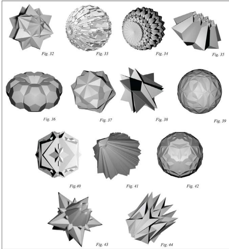
Figura 32: Sabik (103°, S16°); Figura 33: Elnath (278°, N29°); Figura 34: Pollux (244°, N28°); Figura 35: Fomalhaut (16°, S30°); Figura 36: Alkaid (153°, N49°); Figura 37: Alhair (63°, N9°); Figura 38: Dubhe (194°, N62°); Figura 39: Gienah Garab (176°, S17°); Figura 40: Rigil Kentaurus (140°, S60°); Figura 41: Markab (114°, N15°); Figura 42: Alnilam (76°, S1°); Figura 43: Capella (281°, N46°); Figura 44: Etamini (91°, N51°)
