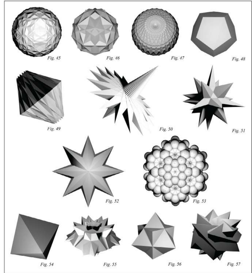
Figura 45: Canopus (264°, S52°); Figura 46: Mirfak (309°, N50°); Figura 47: Alphecca (126°, N27°); Figura 48: Deneb Kaitos (50°, N45°); Figura 49: Hamal (329°, N23°); Figura 50: Menkar (314°, N4°); Figura 51: Ras Alhague (97°, N12°); Figura 51: Alpheratz (358°, N29°); Figura 52: Schedar (350°, N56°); Figura 53: Al- phard (218°, S9°); Figura 54: Avior (234°, S60°); Figura 55: Procyon (245°, N5°); Figura 56: Diphia (349°, S18°); Figura 57: Atria (108°, S69°)
