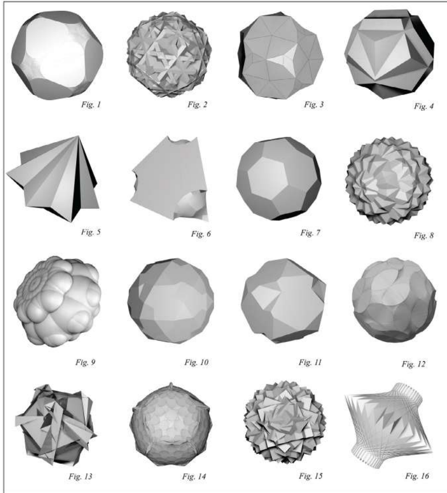
Figura 1: Acamar (316°, S40°); Figura 2: Rigel (282°, S8°); Figura 3: Alioth (167°, N56°); Figura 4: Aldebarán (291°, N16°); Figura 5: Antares (113°, S26°); Figura 6: Menkar (314°, N4°); Figura 7: Kaus Australis (84°, N34°); Figura 8: Enif (34°, N10°); Figura 9: Bellatrix (279°, N6°); Figura 10: Achernar (336°, S57°); Figura 11: Shaula (97°, S37°); Figura 12: Miaplacidus (221°, S70°); Figura 13: Zubenelgenubi (138°, S16°); Figura 14: Peacock (54°, S57°); Figura 15: Vega (81°, N39°); Figura 16: Denebola (183°, N15°).
